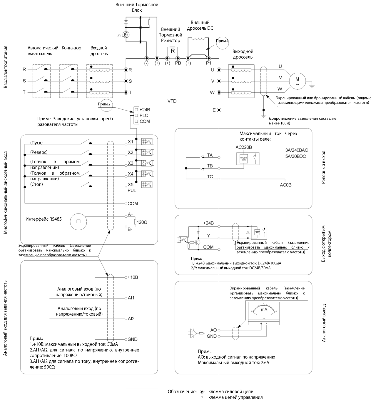
Рис. 3-4 Схема внешних подключений
