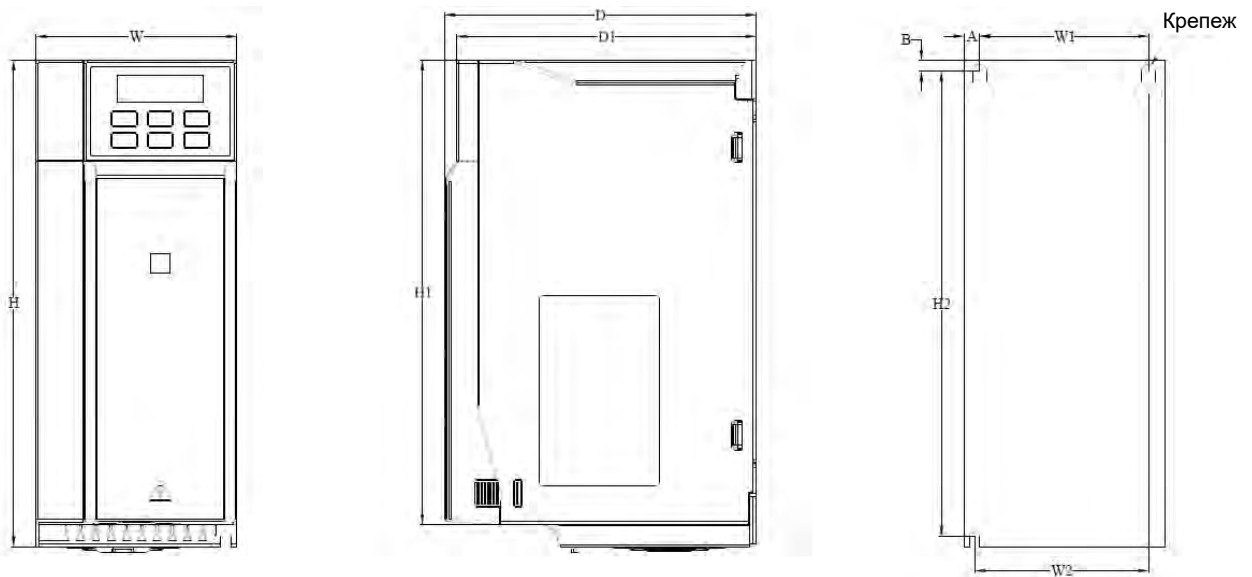
Рис.2-6.2. Чертеж преобразователя частоты типоразмер В2
