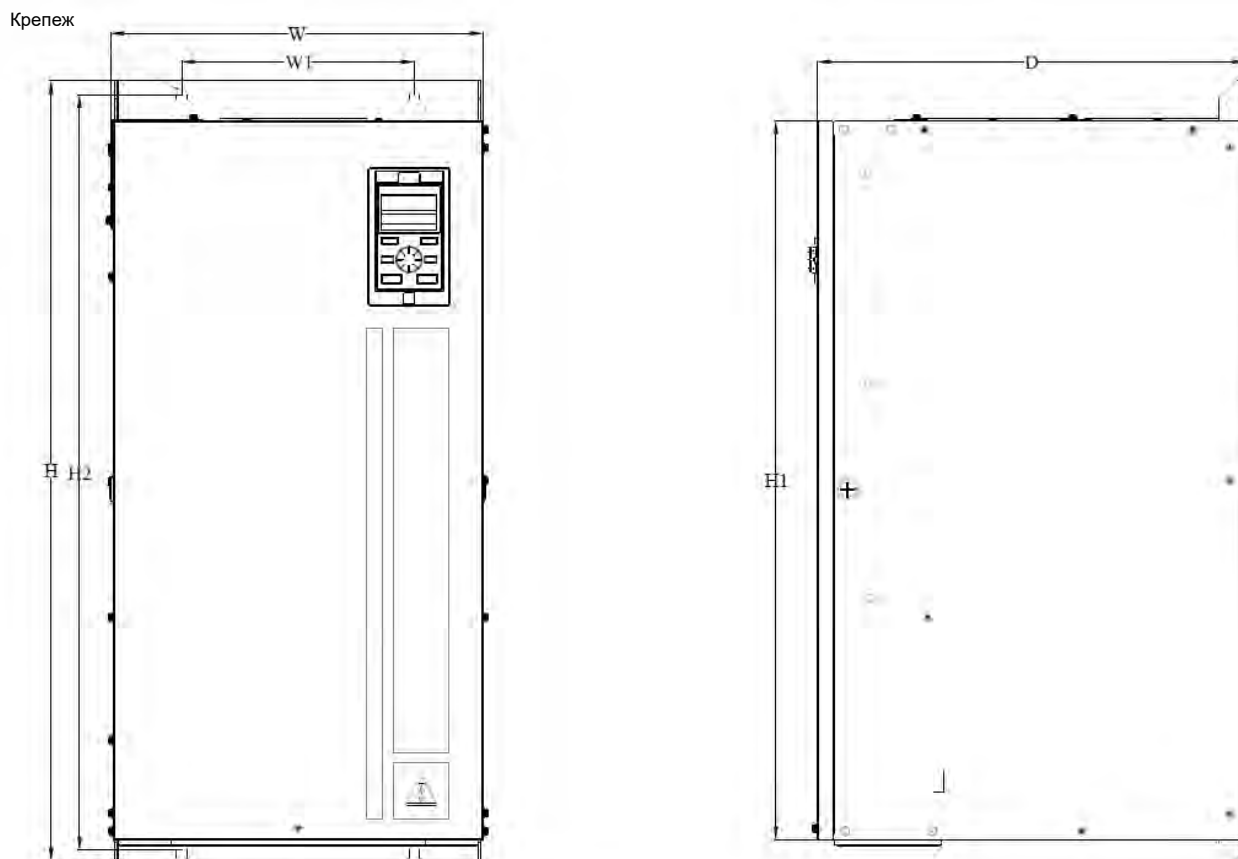
Рис.2-6.7. Чертеж преобразователя частоты типоразмер В7
