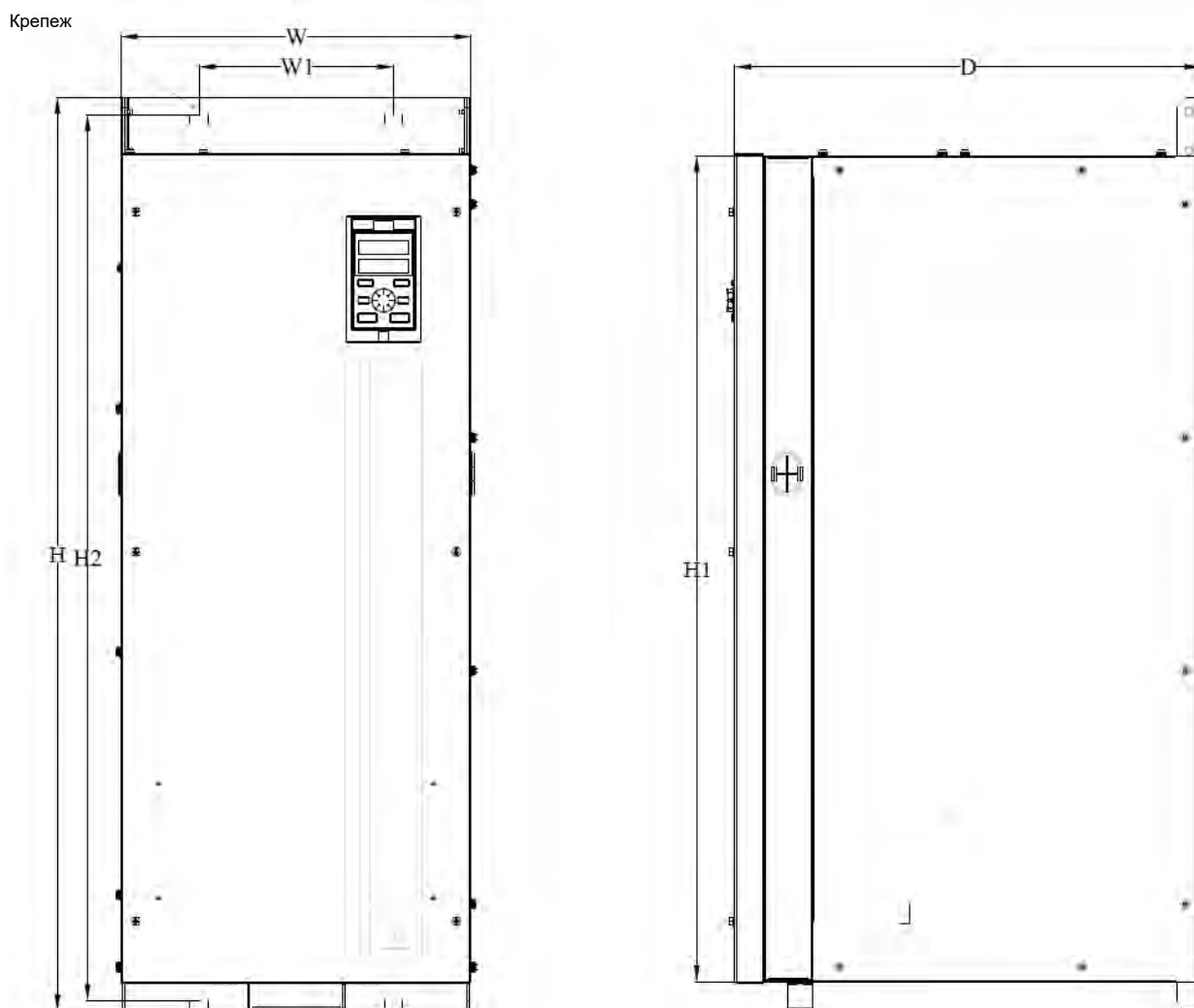
Рис.2-6.8. Чертеж преобразователя частоты типоразмер В8
