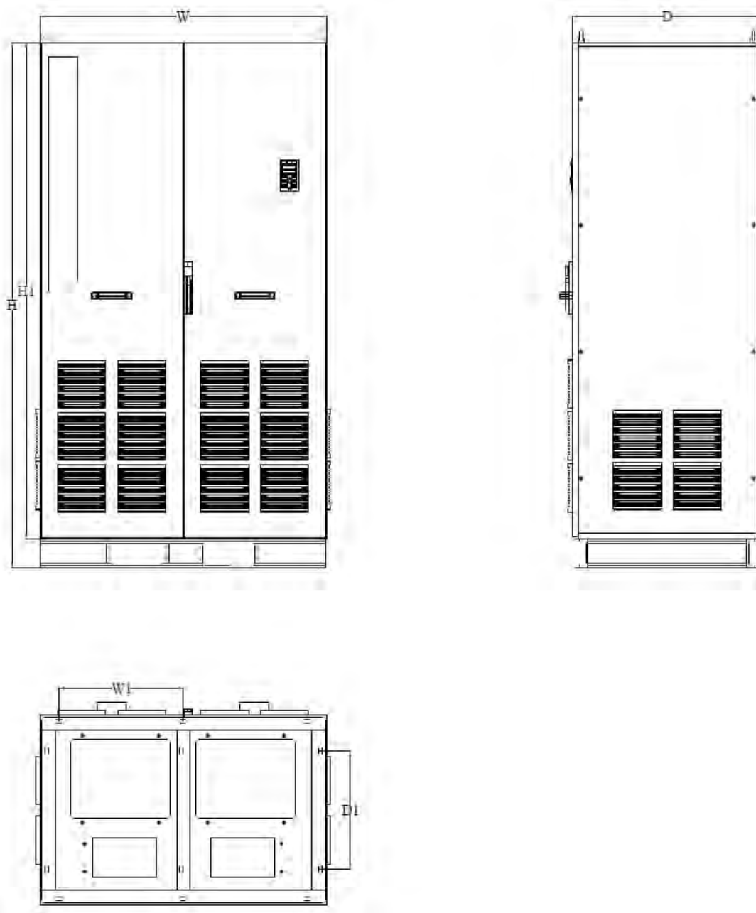
Рис.2-6.12. Чертеж преобразователя частоты типоразмер В12
