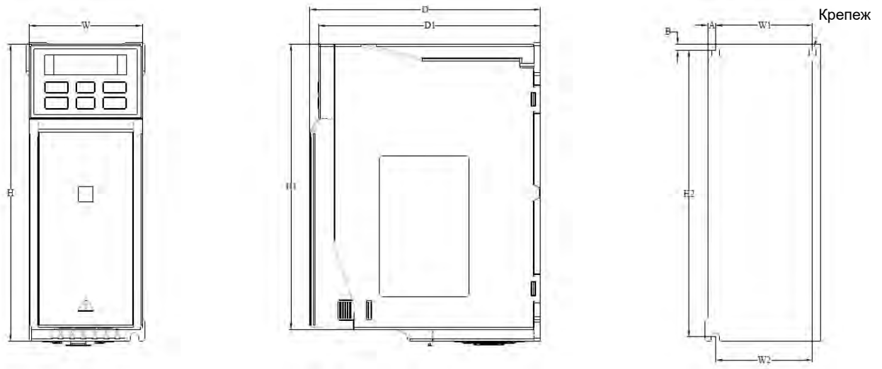
Рис.2-6.1. Чертеж преобразователя частоты типоразмер В1
