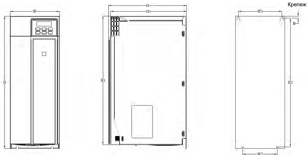
Рис.2-6.4. Чертеж преобразователя частоты типоразмер В4
