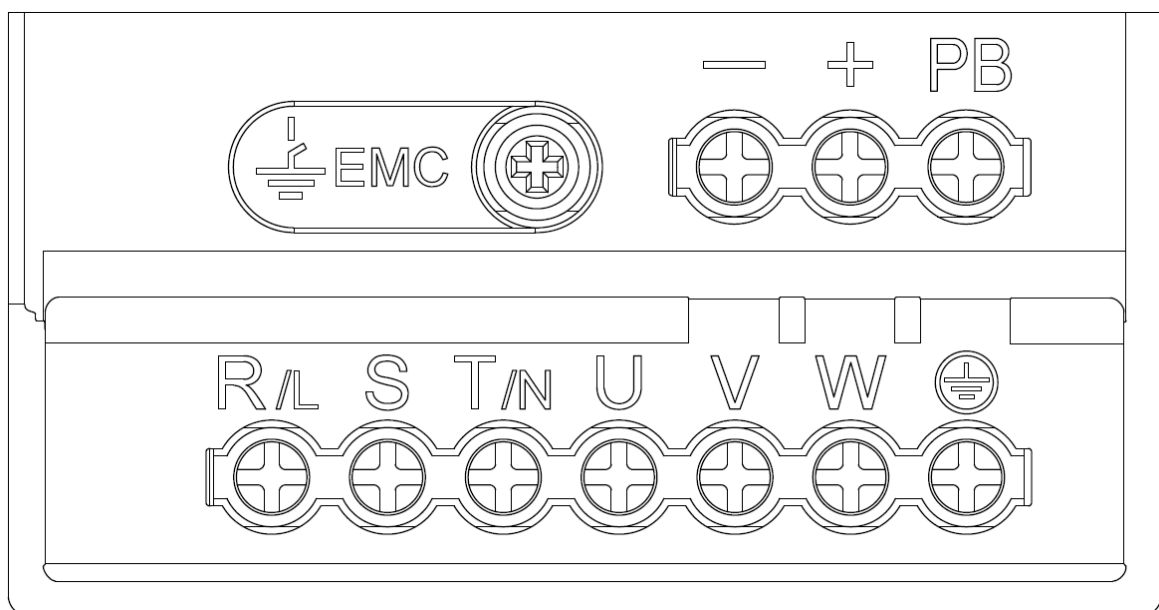
Рис. 3-3.2 Расположение клемм
