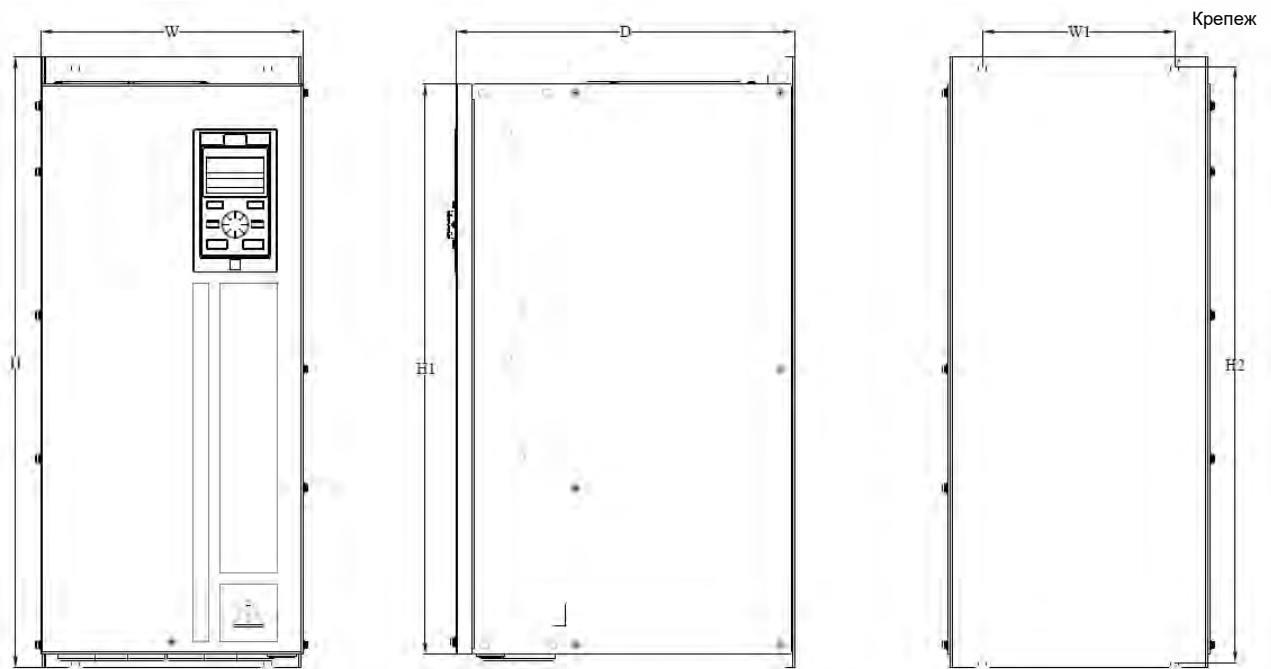
Рис.2-6.6. Чертеж преобразователя частоты типоразмер B6
