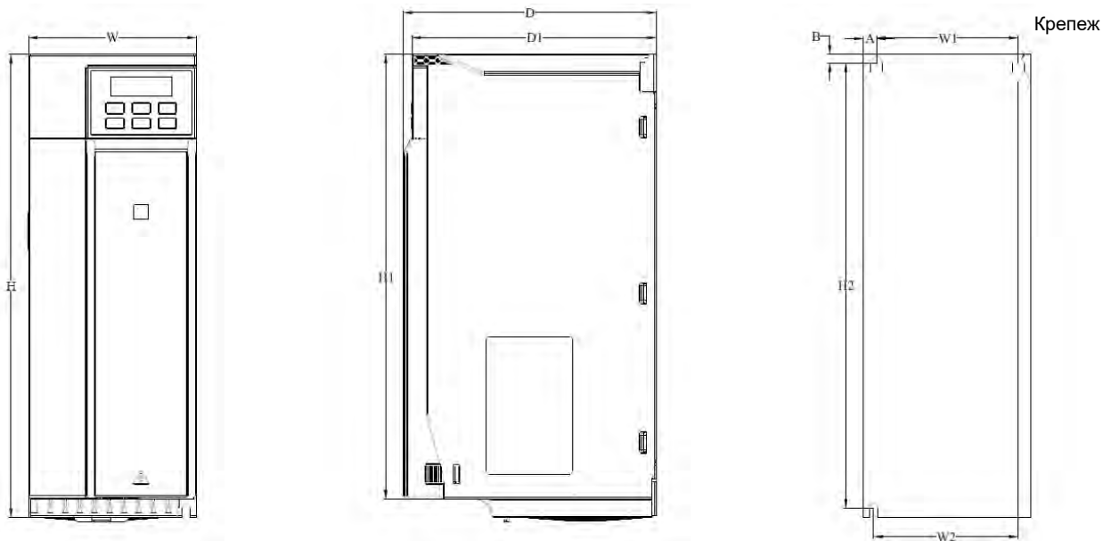
Рис.2-6.3. Чертеж преобразователя частоты типоразмер В3
