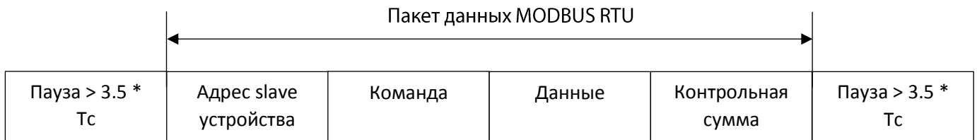
Рис 8-5 Структура пакета MODBUS RTU
