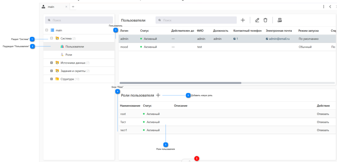
Рисунок 4.8.1 - Общий вид подраздела "Пользователи"
