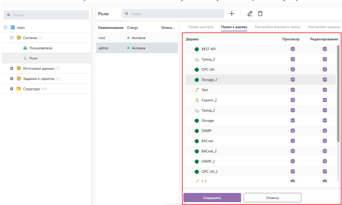
Рисунок 18.1.6 - Окно настройки "Прав доступа к дереву"
