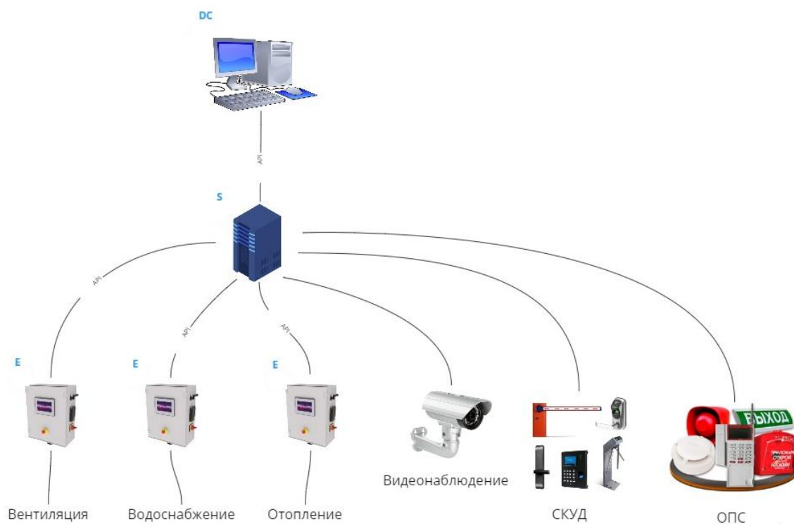
Рисунок 2.2.6 – Архитектурное решение 6
