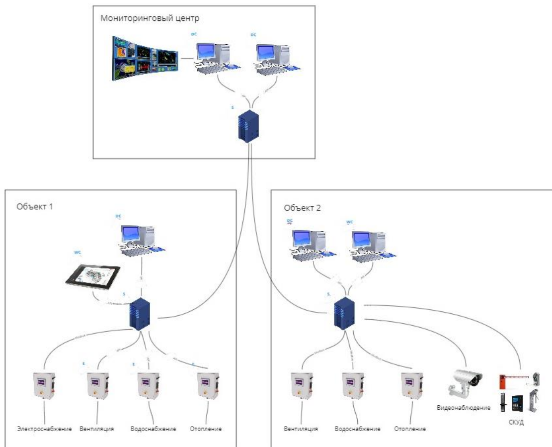
Рисунок 2.2.7 – Архитектурное решение 7
