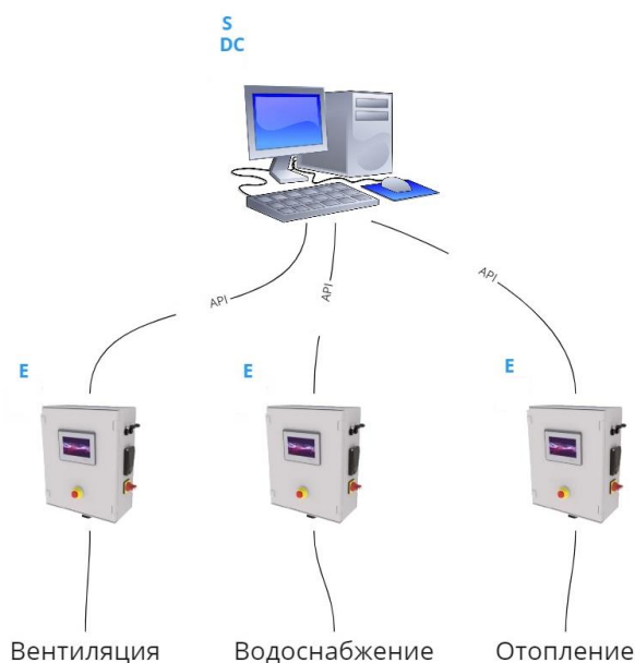
Рисунок 2.2.1 – Архитектурное решение 1
