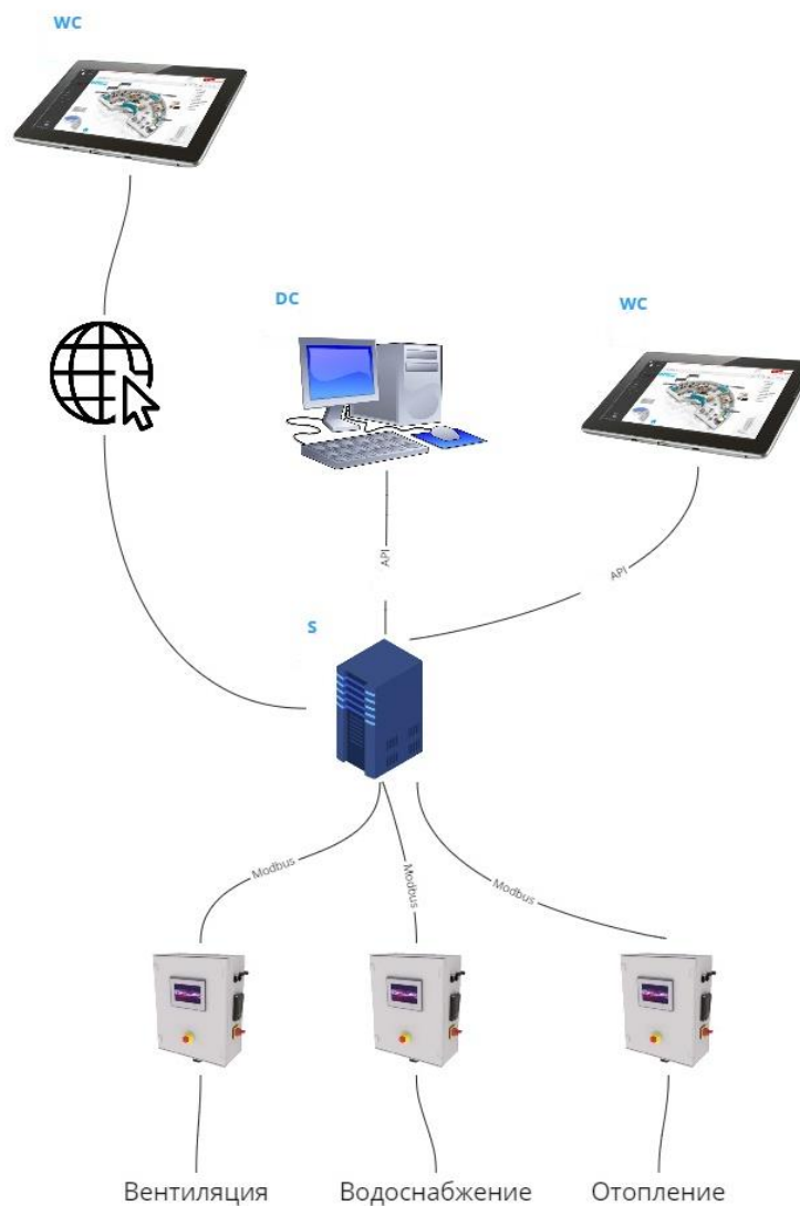
Рисунок 2.2.4 – Архитектурное решение 4
