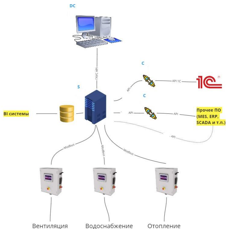
Рисунок 2.2.5 – Архитектурное решение 5
