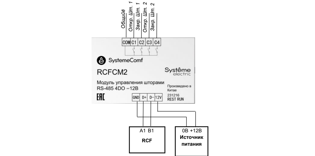
Схема подключения
