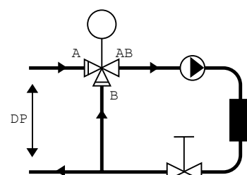
С. Пример системы с циркуляционным насосом.
